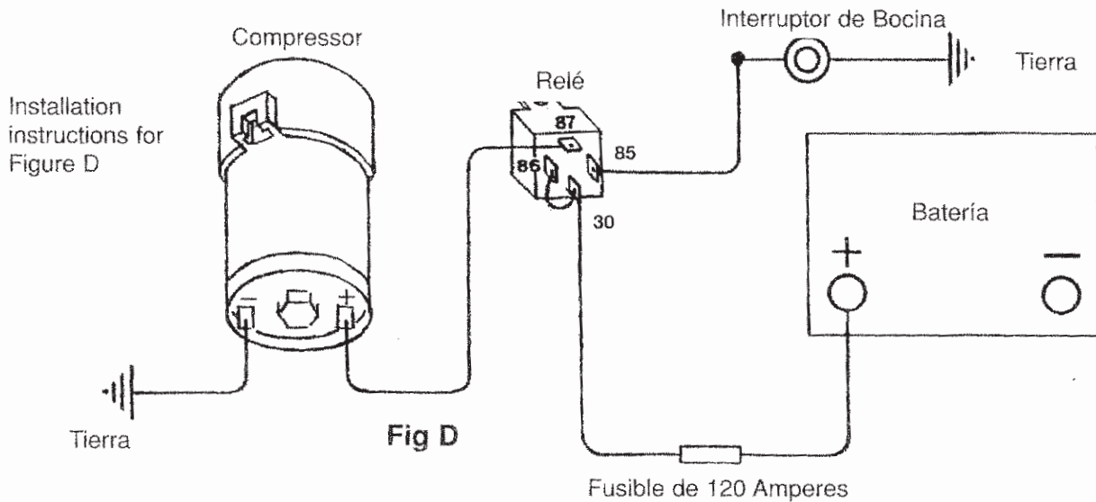
Conexiones Eléctricas
